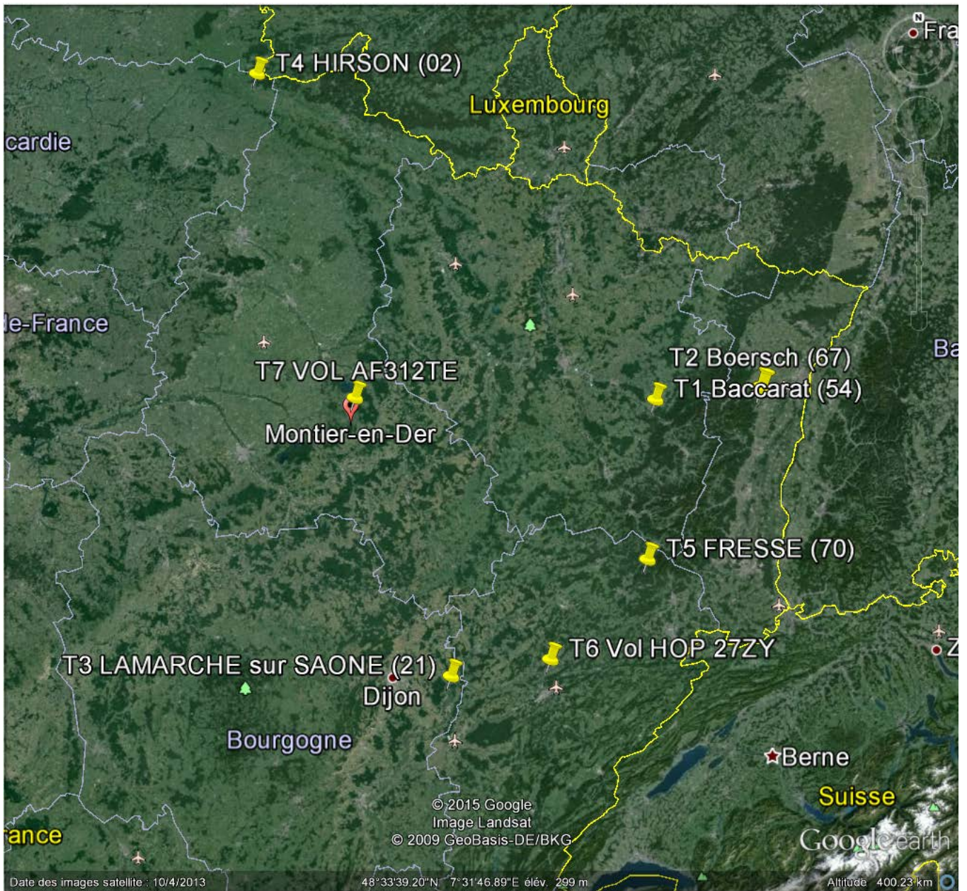
RENTREE ATMOSPHERIQUE (975) 15.03.2015 : positions des témoins.
